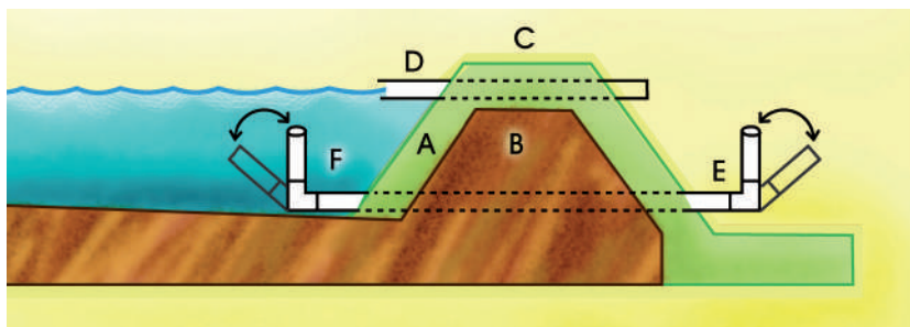
Figura 12. Corte sagital del borde de drenaje. A: bordo con inclinación para evitar deslizamientos, B: corazón de arcilla, C: terraplén, D: tubo de reboso para evitar derrames en temporada de lluvias, E: tubo de drenaje externo con capacidad de inclinarse para ajustar el nivel de vaciado del estanque, F: tubo de drenaje interno con capacidad de inclinarse para ajustar el nivel de vaciado del estanque.
